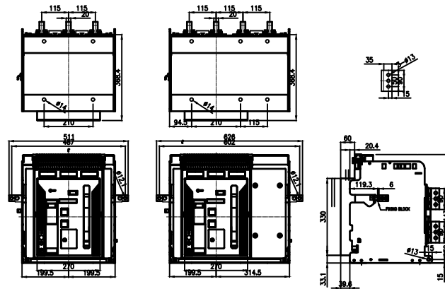
HGN(S) B32 VERTICAL EXTRAIBLE
