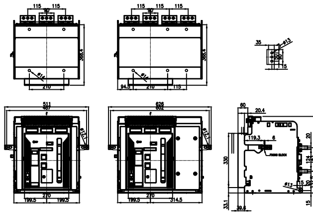
HGN(S) B32 HORIZONTAL EXTRAIBLE
