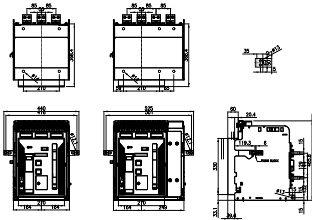
HGN(S) A06~16 HORIZONTAL EXTRAIBLE
